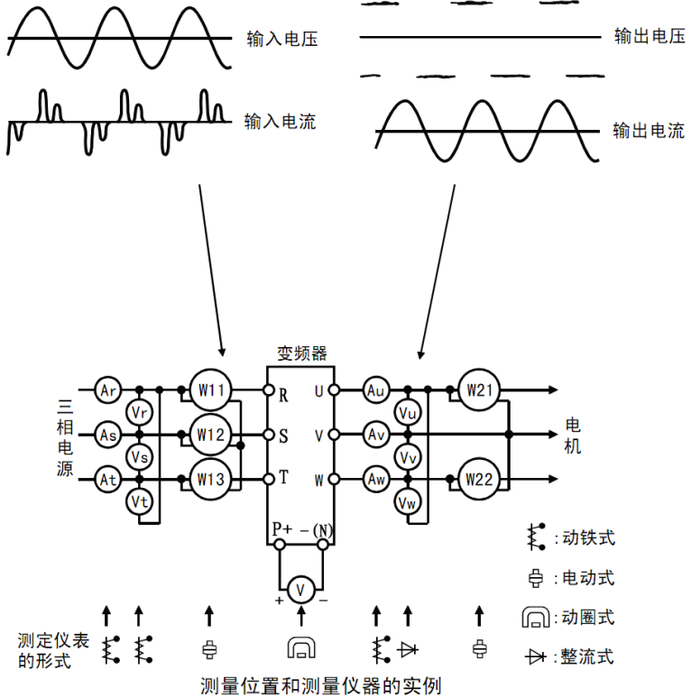
图 4-13 测量示意图
