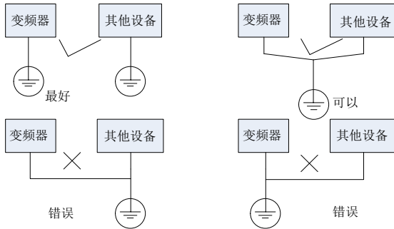
图 4-18 接地示意图
