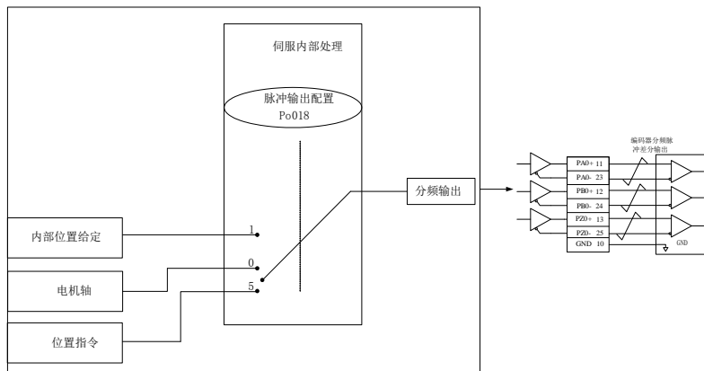
图 7.2.5 分频输出框架图
