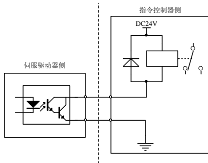
图 4.3.11 继电器输出接口正确电路示意图
