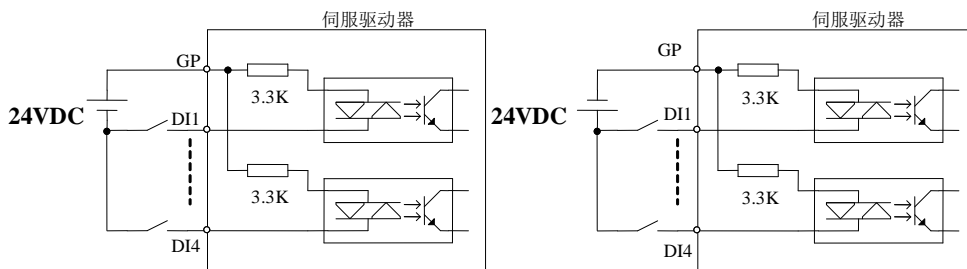
图 4.3.9 无源接点接口电路
