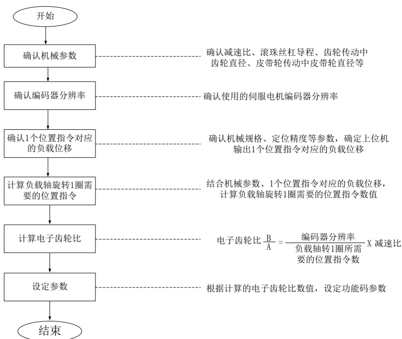
图 7.2.1 电子齿轮比设置步骤流程图
