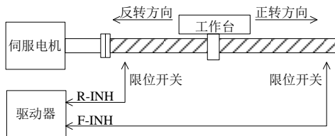
图 7.1.5 超程保护限位开关设置示意图
