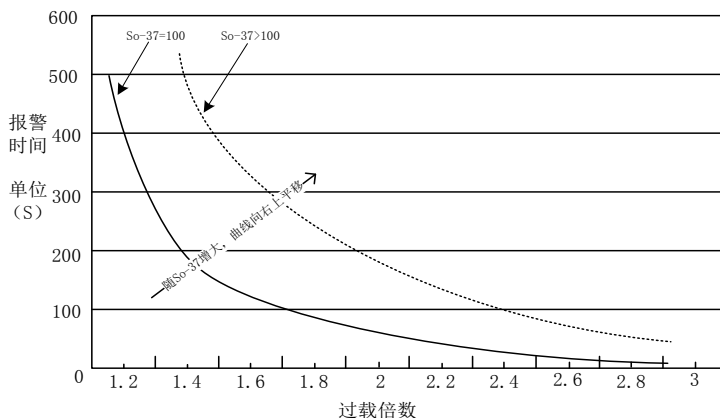
图 7.3.1 电机过载曲线与报警时间曲线图
