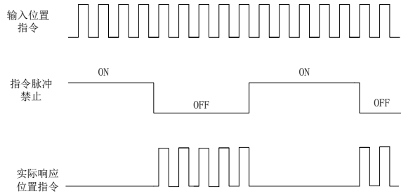
图 7.2.4 位置指令禁止时序图
