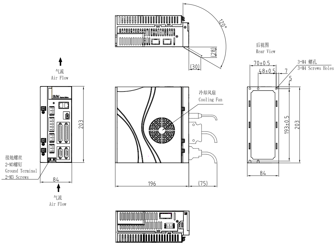
图 3.1.3 伺服驱动器结构尺寸
