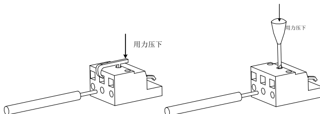
图 4.1.4 主电路端子使用方法
