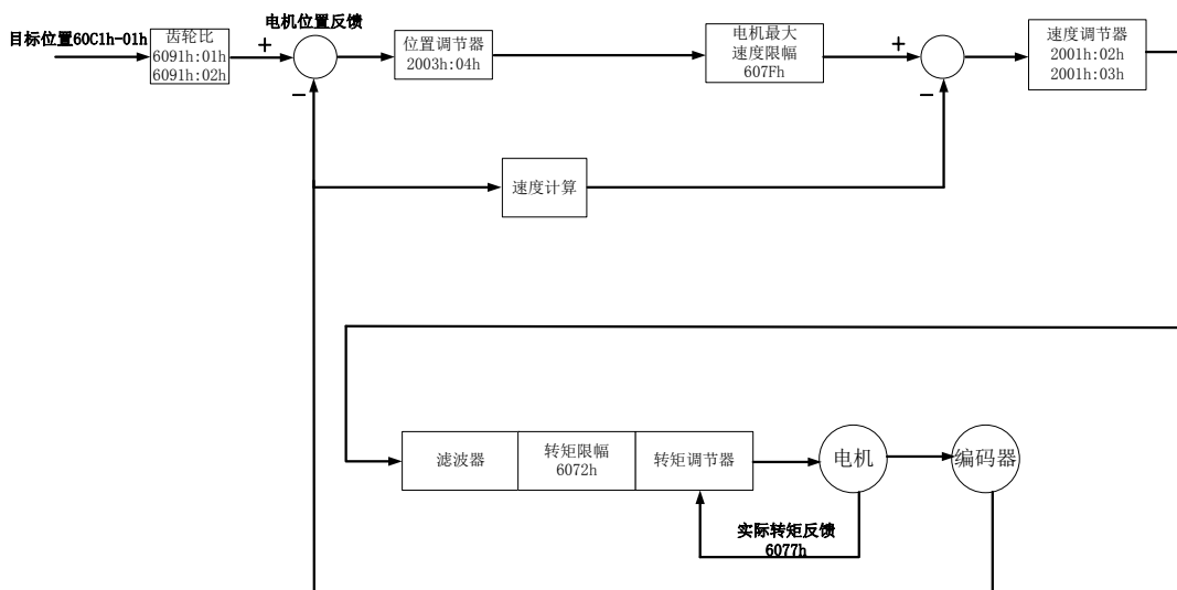
图 7.6.1 周期同步位置 ( ) 控制框图
