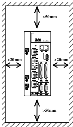
图 3.1.1 典型最小安装尺寸示意图
