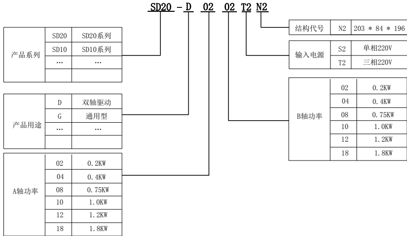
图 2.1.1 伺服驱动器命名规则
