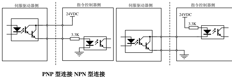
图 4.3.12 光电耦合器输出接口电路
