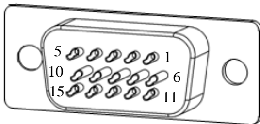
图 4.2.1 绝对值型编码器端子排列示意图
