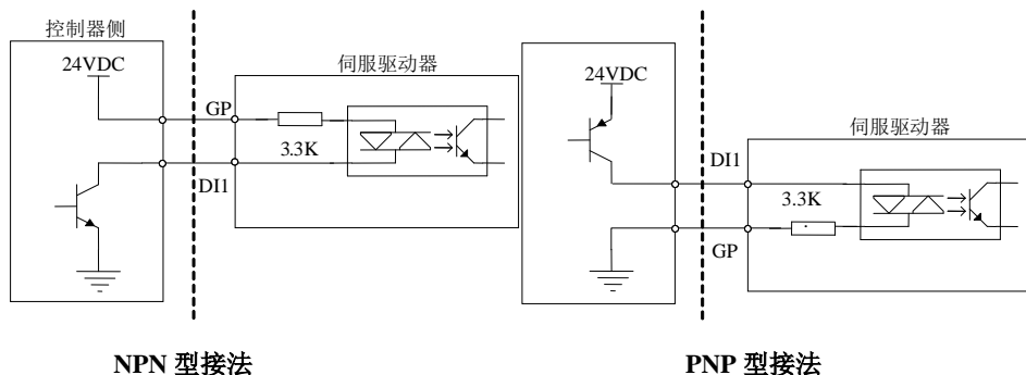
图 4.3.10 有源接点接口电路
