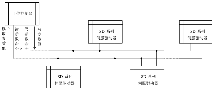
图 6.4.1 现场总线的连接
