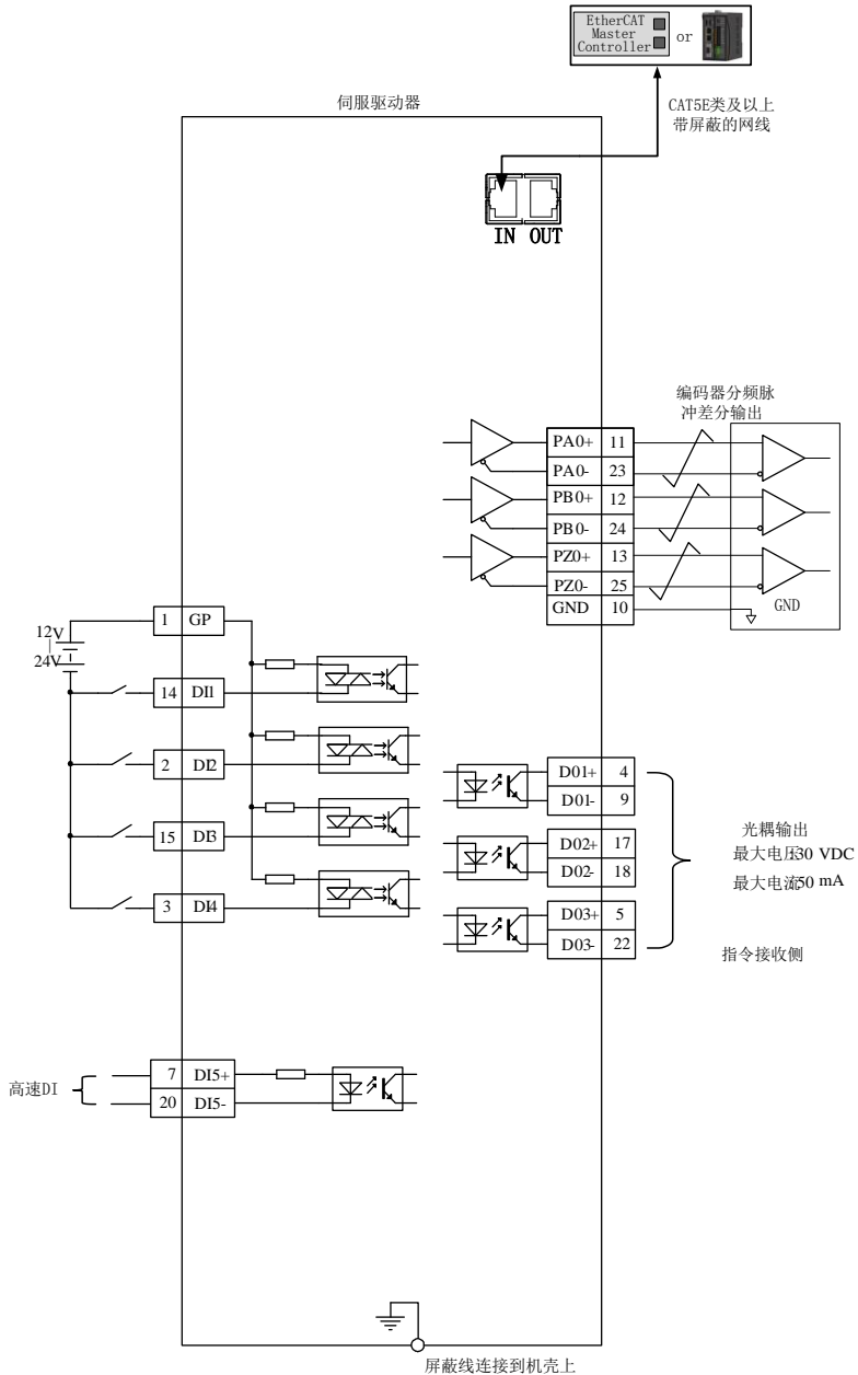
图 4.3.1 三种模式下接线示意图
