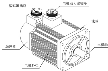
图 2.2.5 伺服电机各部分名称
