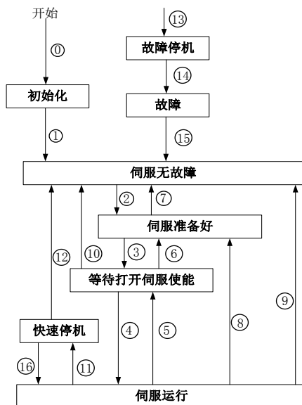
图 7.2.1 CiA402 状态机切换图
