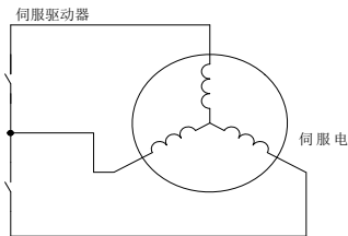
图 7.1.9 动态制动的示意图
