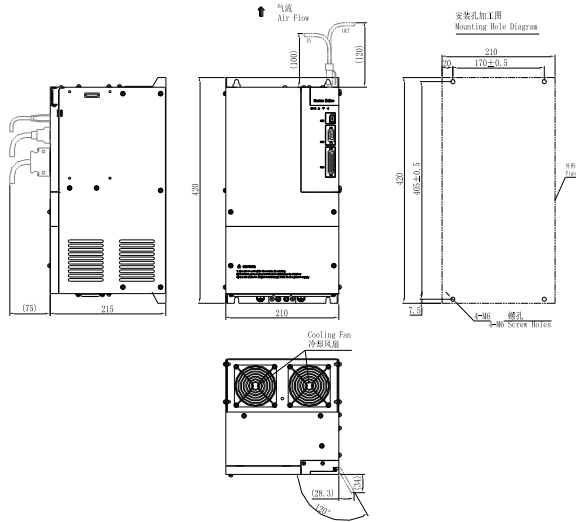
图 3.1.9 伺服驱动器结构尺寸 7
