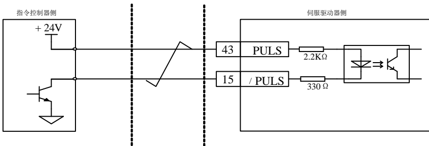
图 4.3.6 24V 集电极开路脉冲输入接口电路
