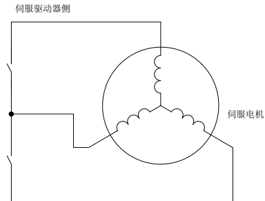
图 7.1.9 动态制动的示意图
