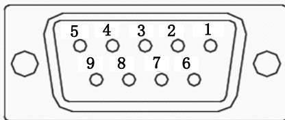
图 4.2.1 绝对值型编码器端子排列示意图
