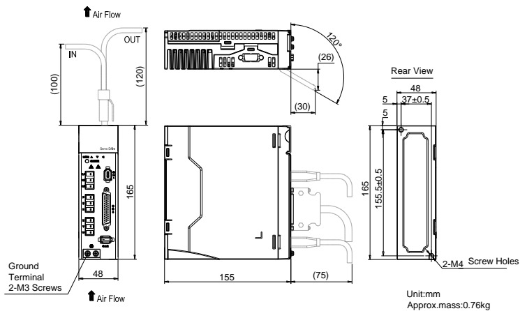
图 3.1.3 伺服驱动器结构尺寸 1
