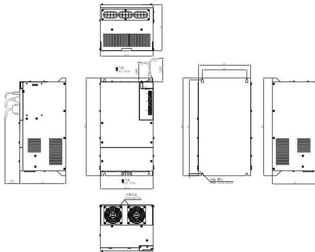
图 3.1.10 伺服驱动器结构尺寸 8
