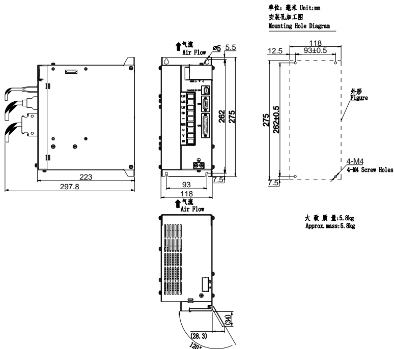
图 3.1.7 伺服驱动器结构尺寸 5
