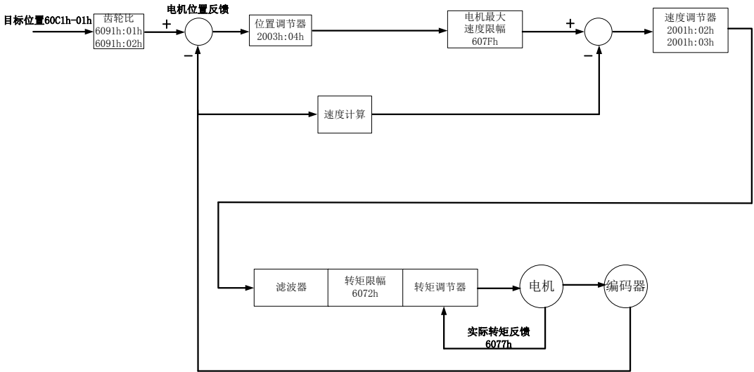
图 7.6.1 位置插补模式 (IP) 控制框图
