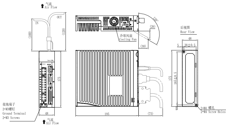
图 3.1.4 伺服驱动器结构尺寸 2
