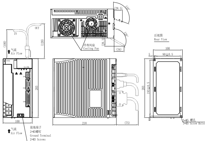
图 3.1.6 伺服驱动器结构尺寸 4
