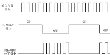
图 7.2.4 位置指令禁止时序图
