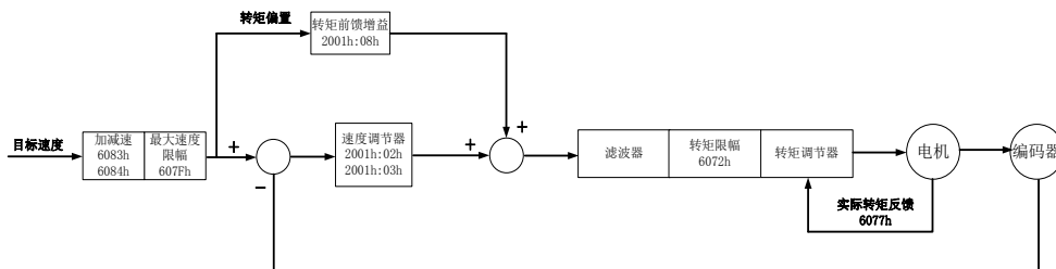
图 7.4.1 轮廓速度模式（PV）控制框图
