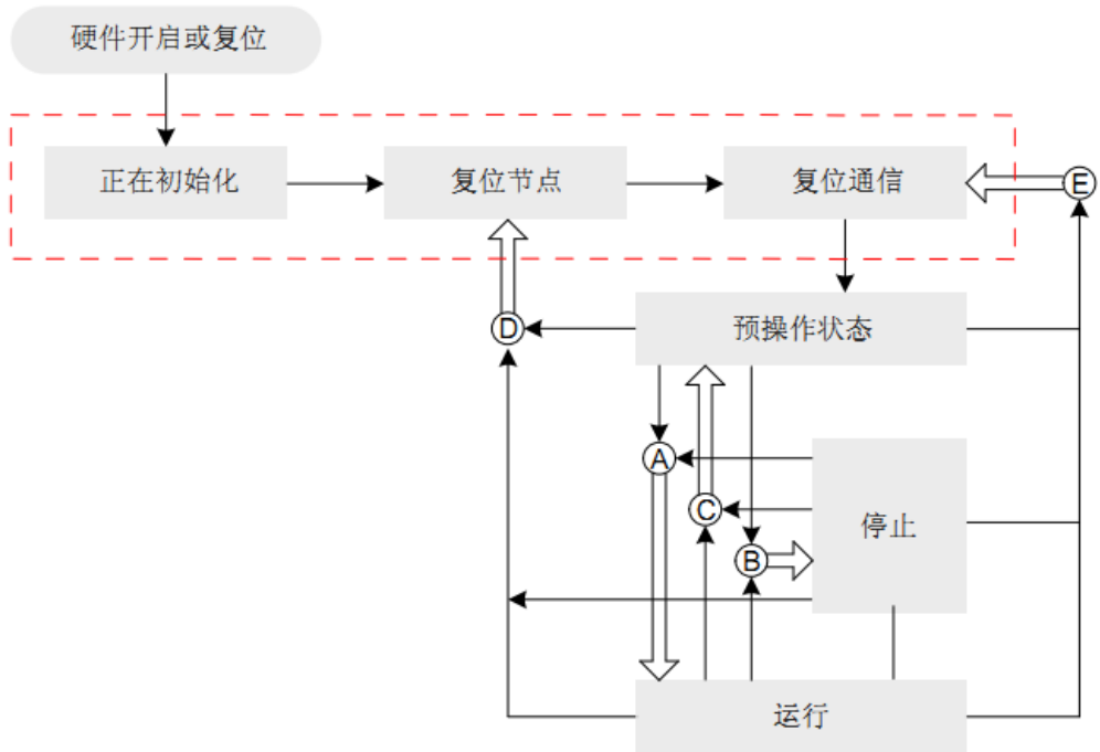
NMT 状态机执行图
