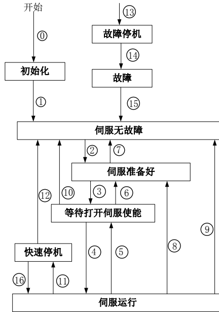
图 7.2.1 CИА402 状态机切换图
