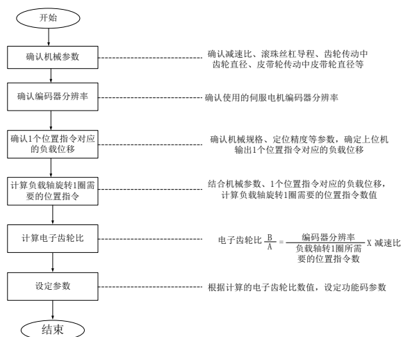
图 7.2.1 电子齿轮比设置步骤流程图
