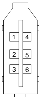
图 4.3.22 通讯口 CN1 插头端子排列顺序图
