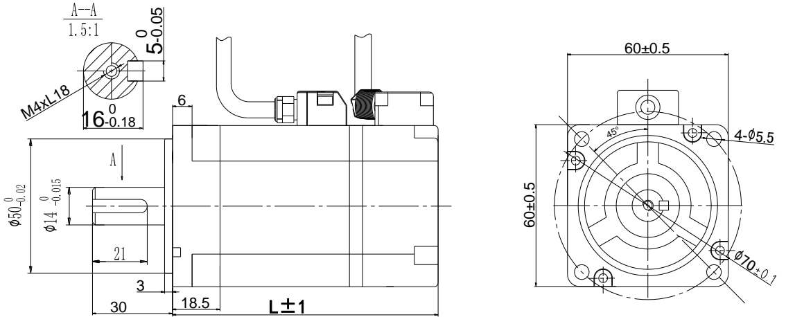
60 法兰五对极伺服电机外形尺寸图
