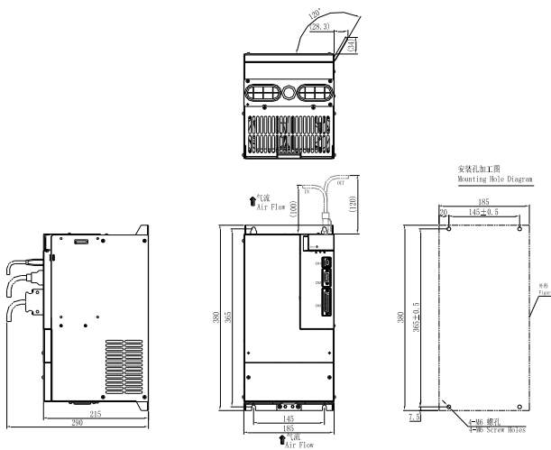
图 3.1.8 伺服驱动器结构尺寸 6
