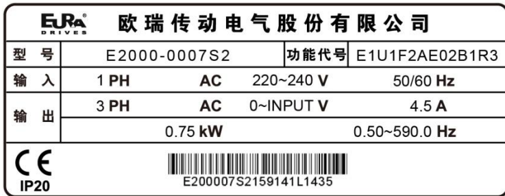
图 2-3 产品铭牌
