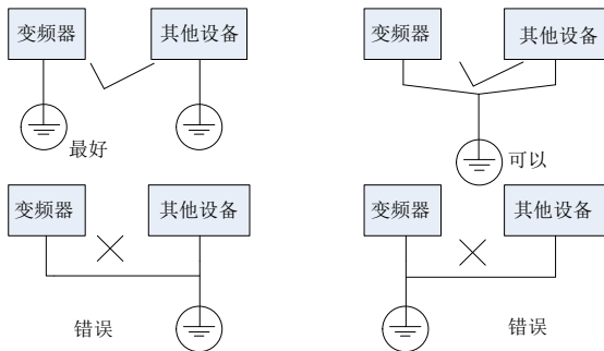
图 4-18 接地示意图
