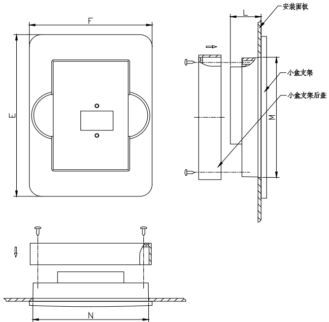
图 3-5 控制面板安装支架结构尺寸示意图
