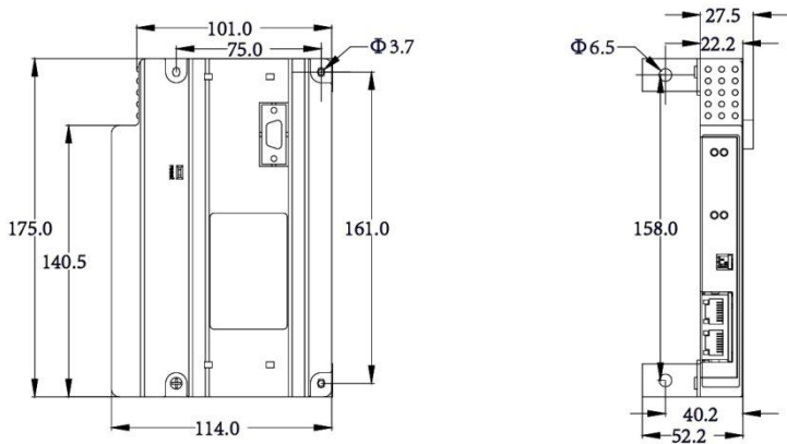
图 10-2 变频器 EtherCAT 总线卡尺寸图
