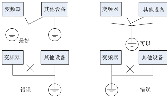
图 4-24 接地示意图
