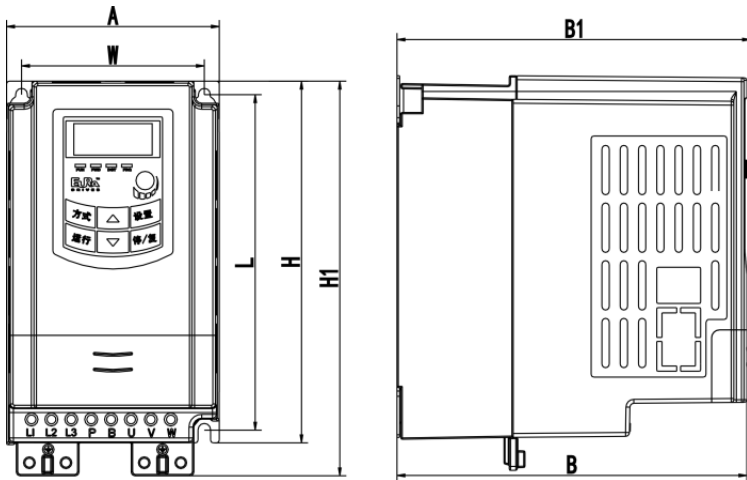
塑壳外形
