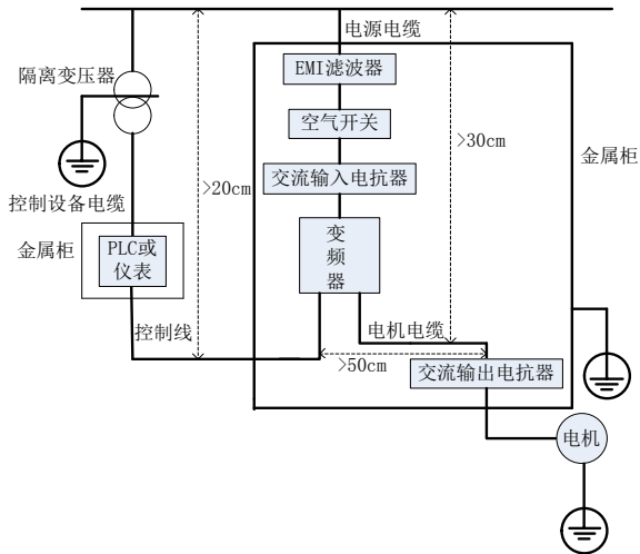
图 4-25 电气安装示意图
