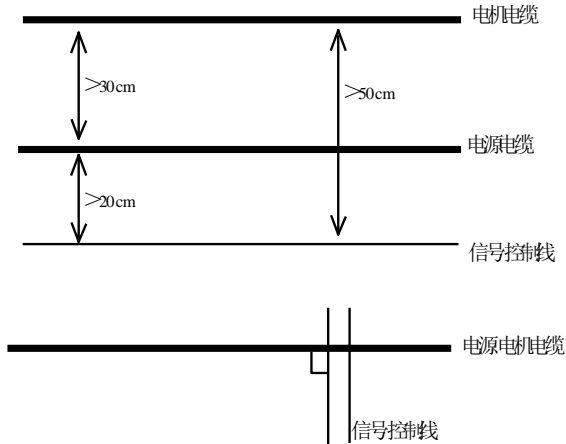
图 4-23 现场配线示意图
