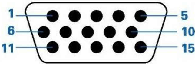
图 10-7 接口引脚图
