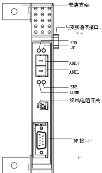
图 10-14 通讯卡外形及结构部件图
