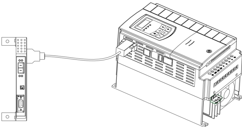
图 10-11 变频器 Profibus 总线卡安装示意图
