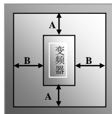
图 4-1 变频器安装示意图
