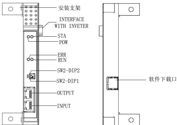
图 10-3 变频器 EtherCAT 总线卡示意图
