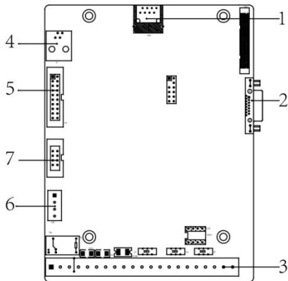
图 2-6 E7 及铁壳接口图
