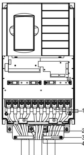
图 4-16 塑壳 (E7) 壁挂功率接线示意图
