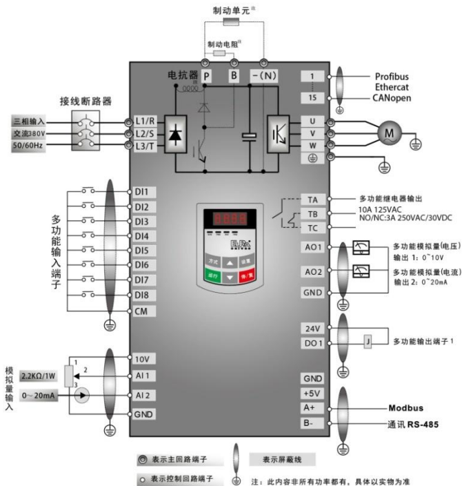
图 4-14 三相变频器标准配线图(NPN 方式)
