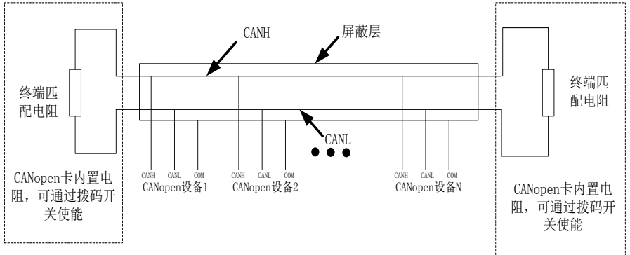
图 10-8 CAN -bus 接线示意图
