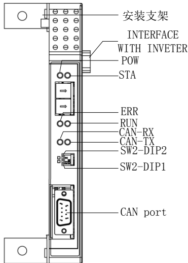
图 10-9 变频器 CANopen 总线卡示意图
