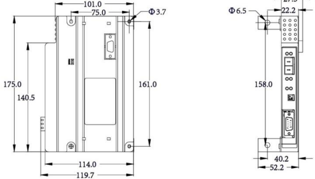
图 10-6 变频器 CANopen 总线卡尺寸图
