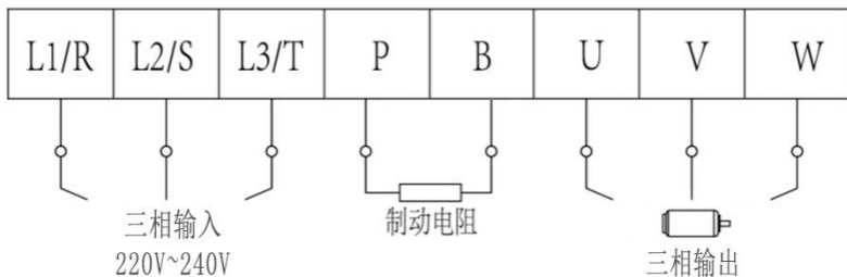
图 4-3 端子示意图
