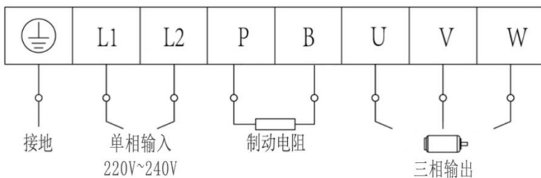
图 4-2 端子示意图
