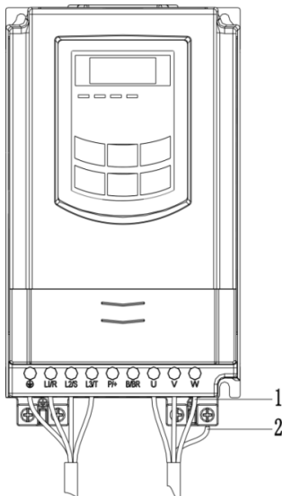
图 4-15 塑壳(E1~E6)壁挂功率接线示意图
