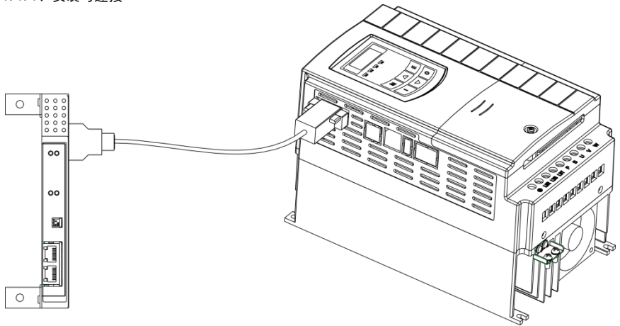
图 10-1 变频器 EtherCAT 总线卡安装示意图
