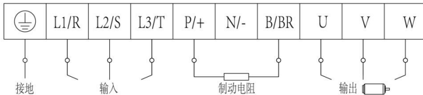
图 4-5 端子示意图
