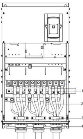
图 4-17 金属壁挂功率接线示意图
