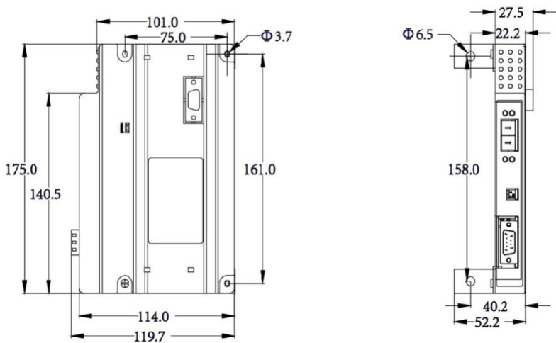
图 10-12 变频器 Profibus 总线卡外观尺寸图
