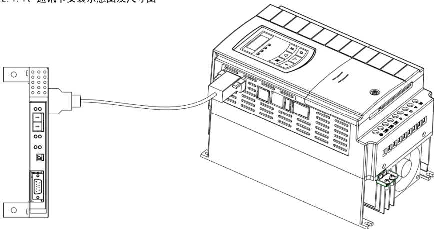
图 10-5 变频器 CANopen 总线卡安装示意图
