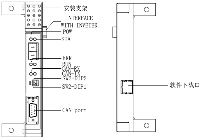
图 10-10 接口说明示意图
