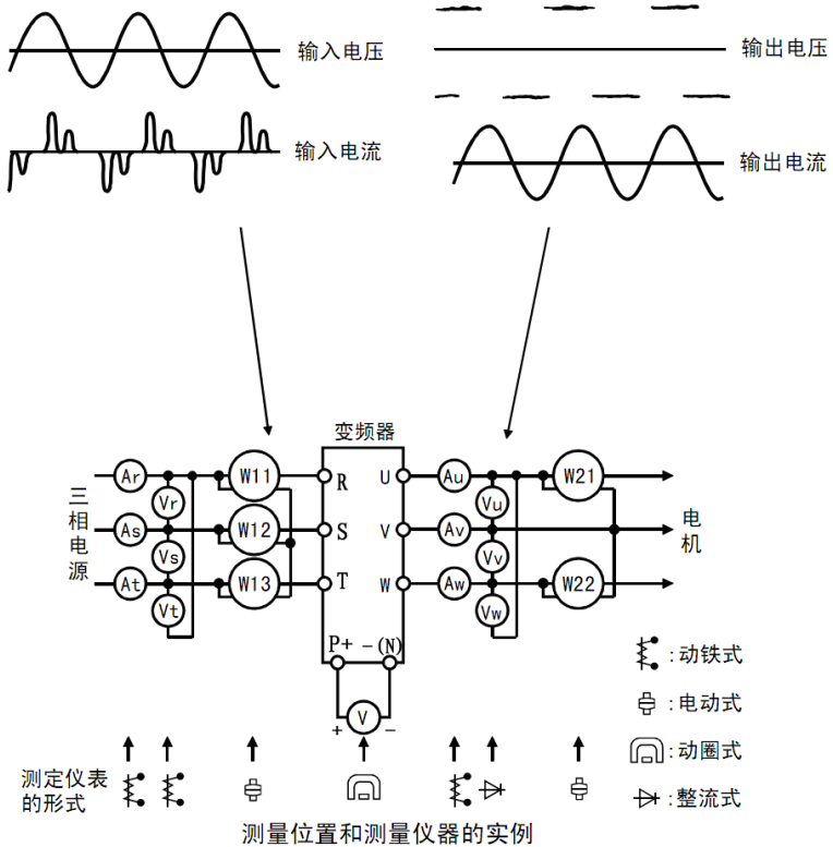
图 4-13 测量示意图
