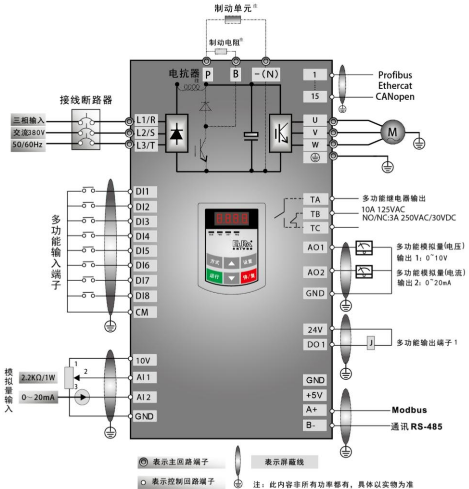
图 2-1 三相变频器标准配线图 (NPN 方式)
