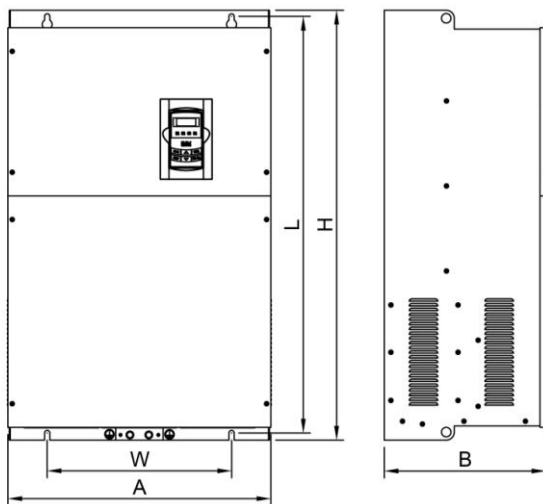
塑壳外形
