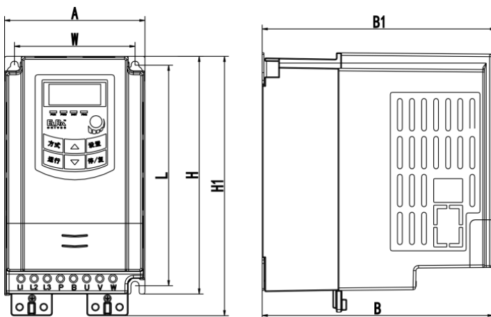
塑壳外形
