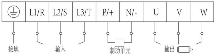
图 4-5 端子示意图
