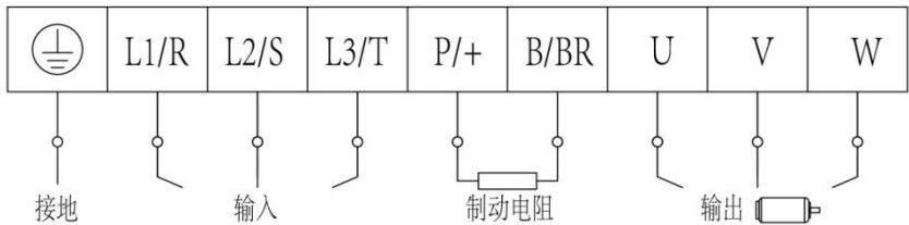
图 4-2 端子示意图
