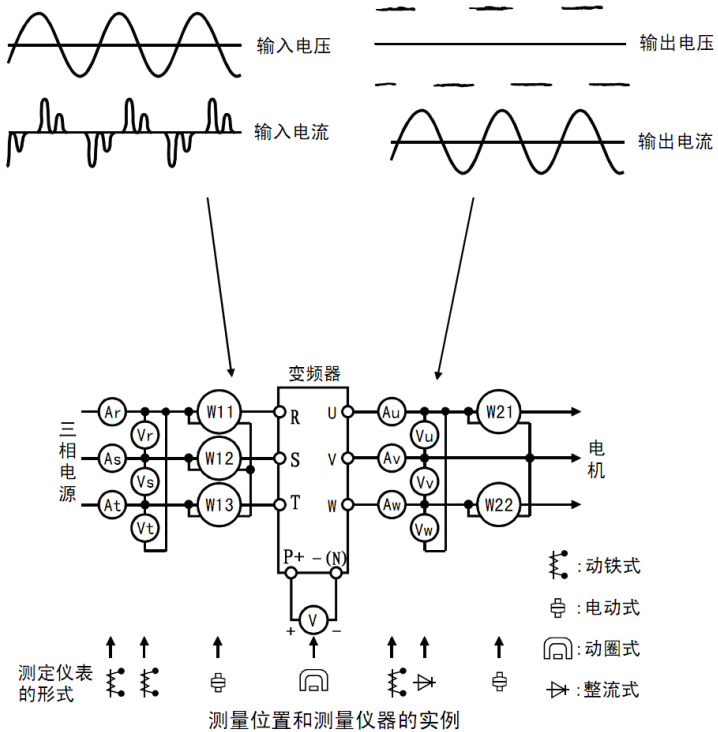
图 4-11 测量示意图
