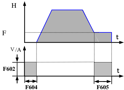
图 6-16 直流制动
