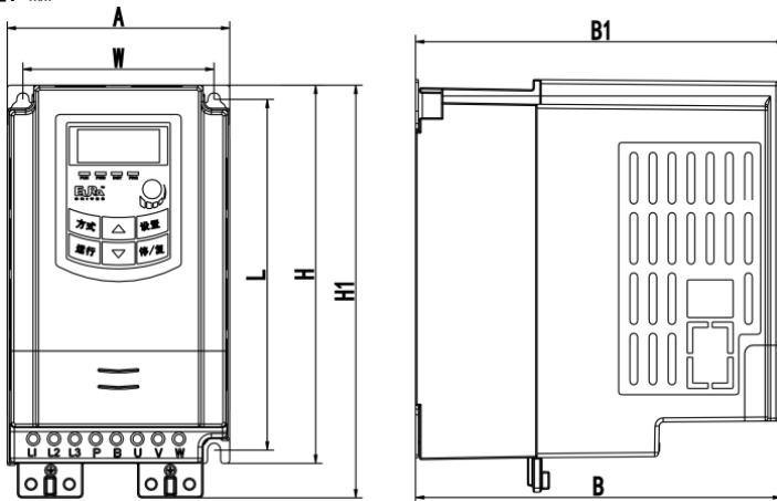
塑壳外形
