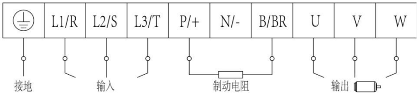
图 4-3 端子示意图
