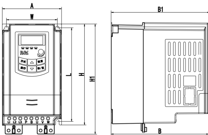
塑壳外形
