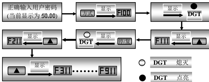
图 3-6 功能码区内和区间切换
