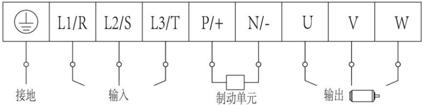
图 4-5 端子示意图
