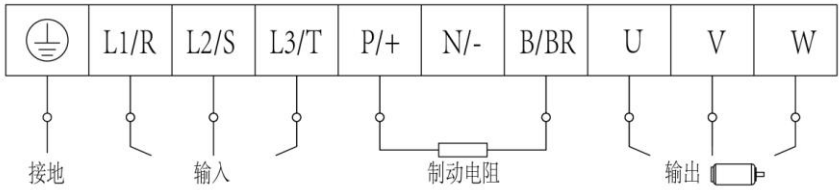
图 4-3 端子示意图
