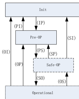
图 6.3.2 EtherCAT 状态机
