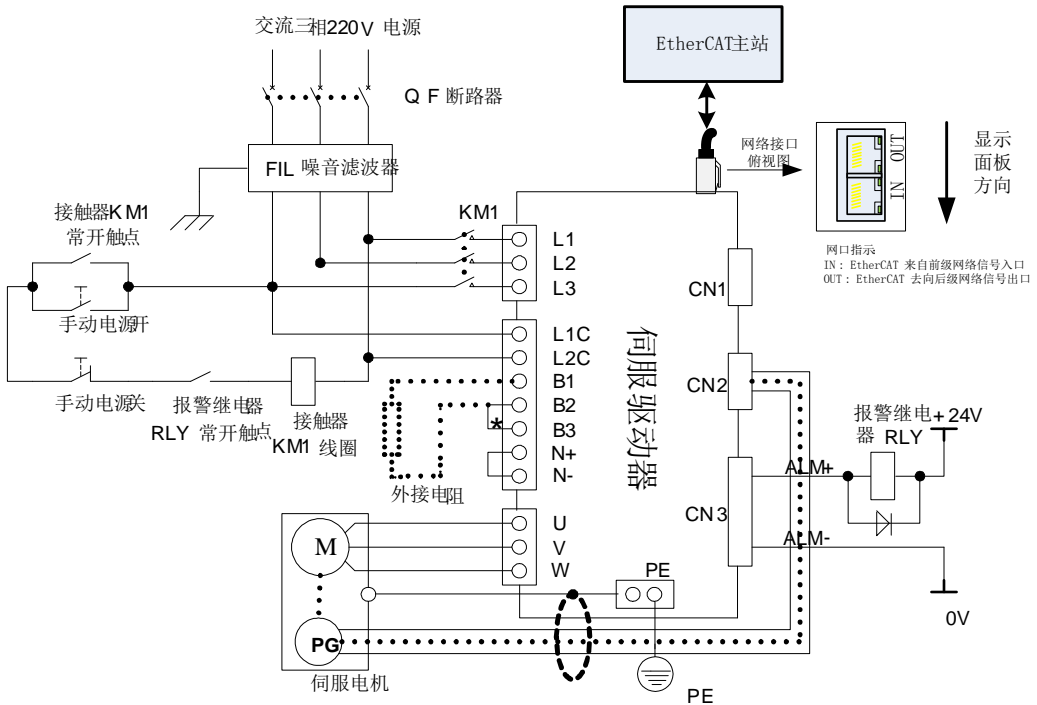
图 4.1.4 220V 驱动器典型主电路配线图
