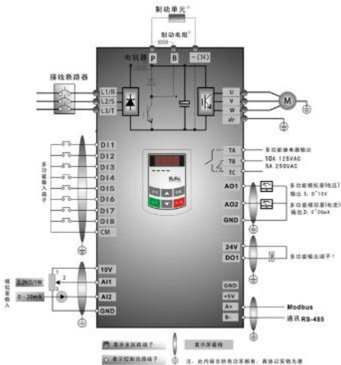
图 4-8 三相变频器标准配线图 (NPN 方式)
