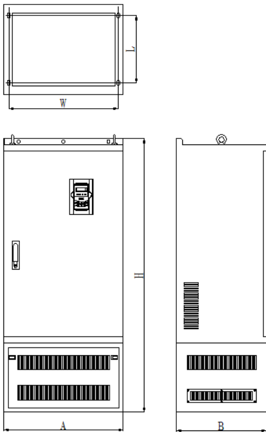
1140V 机壳外形
