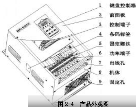
图 2-4 产品外观图
