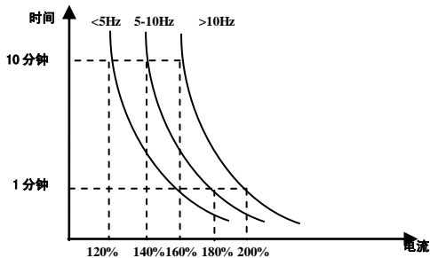
图 6-21 不同频率下的电机过载保护值
