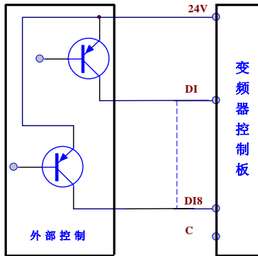
图 4-6 有源共漏极接线方式示意图
