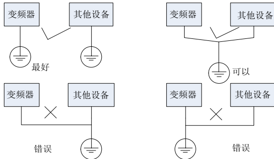
图 4-12 接地示意图
