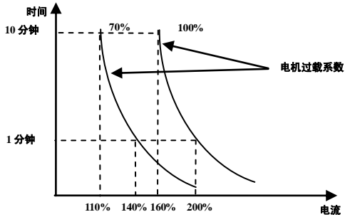
图 6-20 电机过载系数设定
