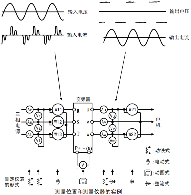
图 4-2 测量示意图
