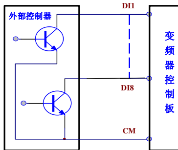
图 4-4 有源共源极接线方式示意图
