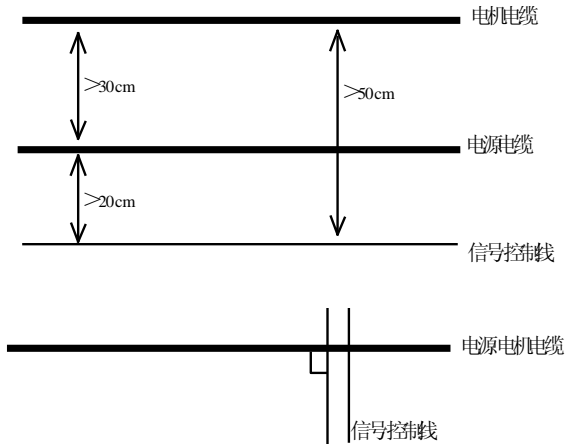
图 4-11 现场配线示意图
