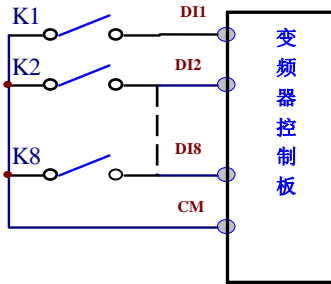
图 4-3 无源共源极接线方式示意图
