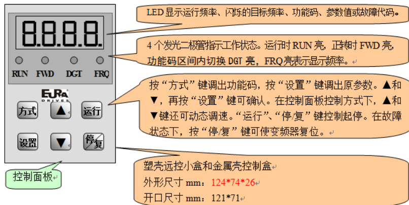
图 3-1 控制面板
