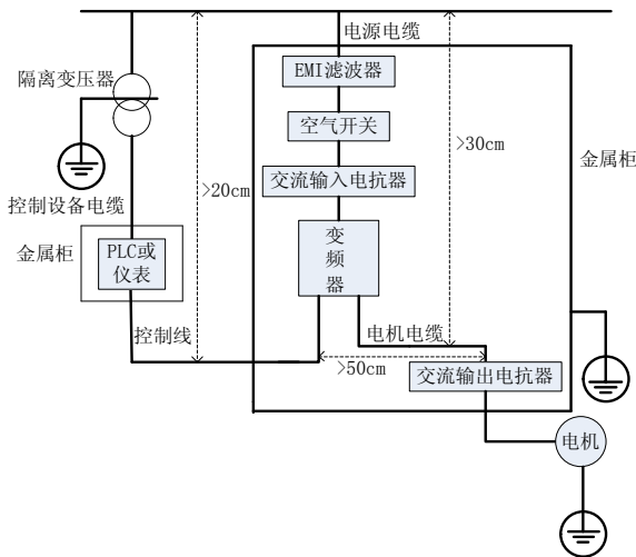
图 4-13 电气安装示意图
