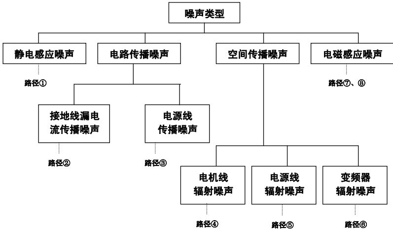
图 4-9 噪声类型图示
