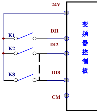
图 4-5 无源共漏极接线方式示意图
