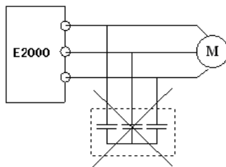
图 1-4 变频器输出端禁止使用电容器
