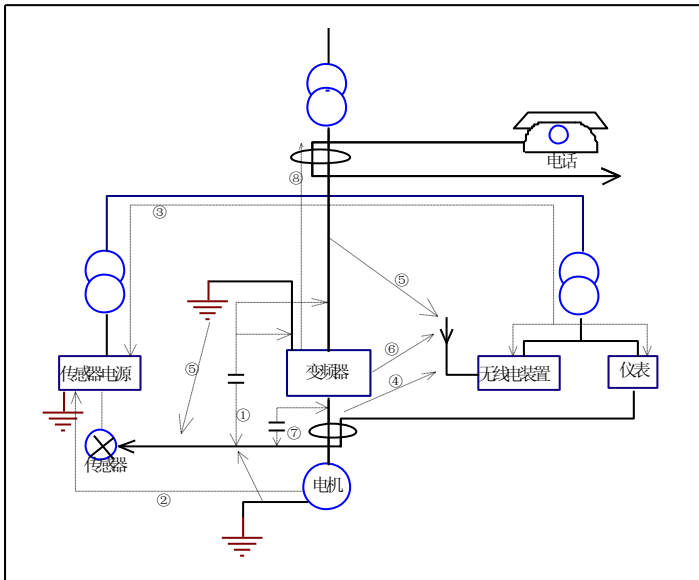
图 4-10 噪声传播途径
