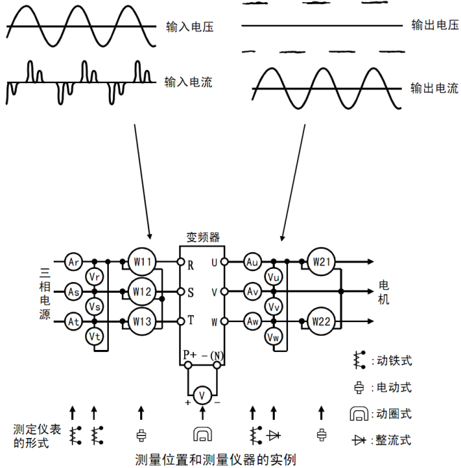
图 4-9 测量示意图
