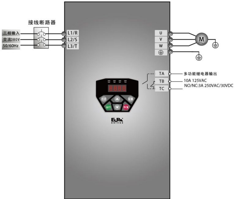
5-1 接线图 1
