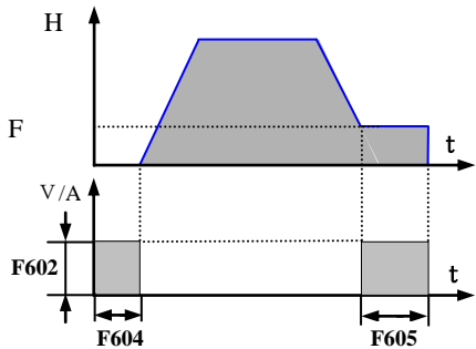
图 6-20 直流制动
