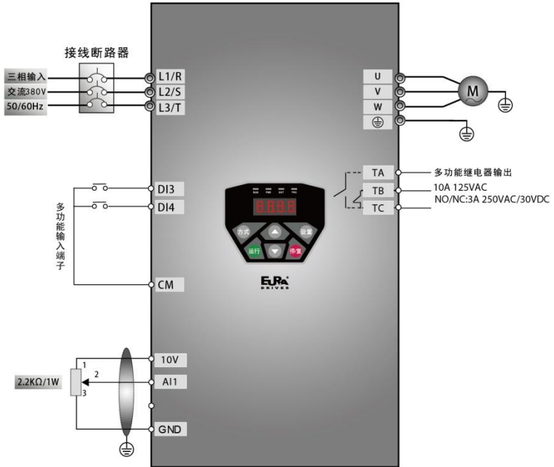
图 5-3 接线图 3
