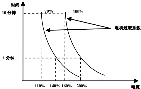
图 6-21 电机过载系数设定
